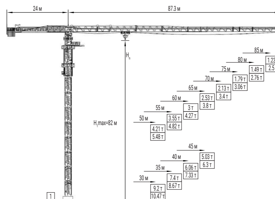
QTZ 600 (8525) – 32t
