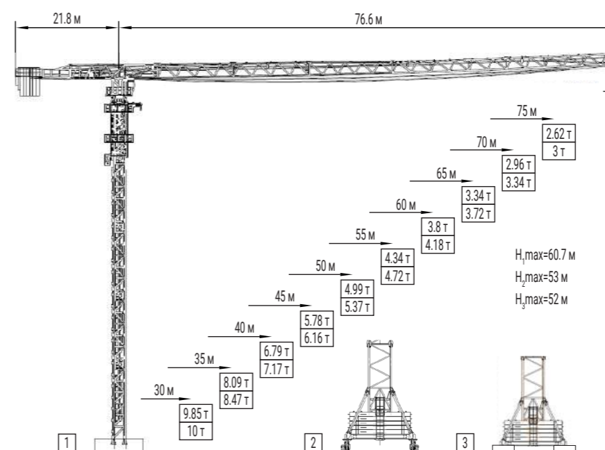
QTZ 250 (7530) – 20t
