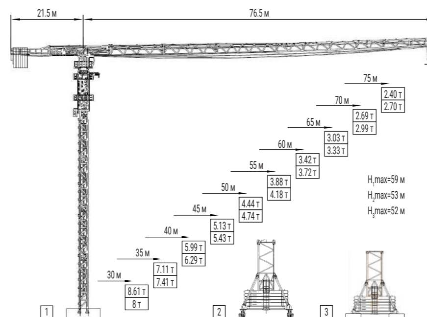
QTZ 250 (7527) – 16t
