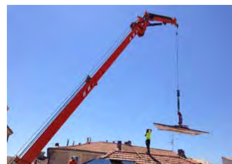
Вакуумный захват
