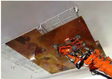
Вакуумный захват
